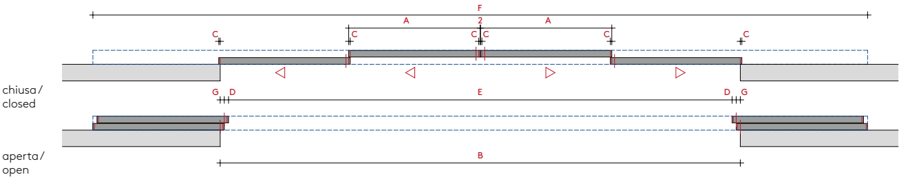
Binario due vie_4 divisori scorrevoli con trascinamento singolo a scomparsa (da entrambi i lati) / Two ways rail_4 sliding partitions with single concealing dragging system (from both sides)
