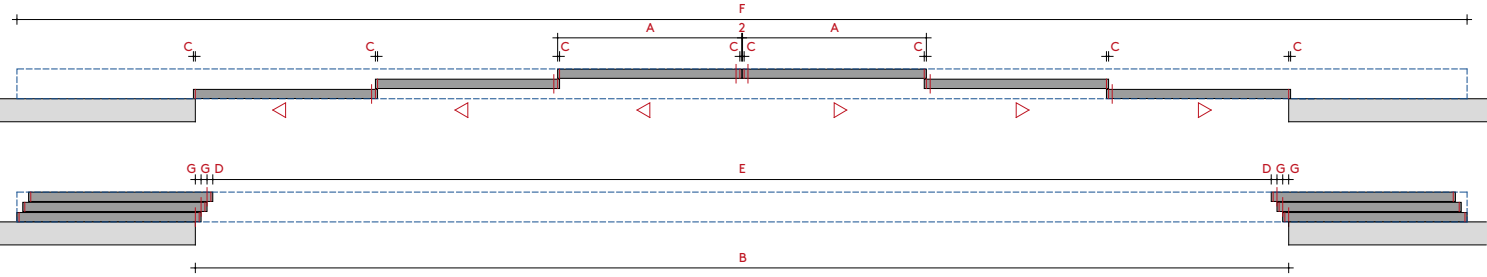
Binario tre vie_6 divisori scorrevoli con trascinamento doppio a scomparsa (da entrambi i lati) / Three ways rail_6 sliding partitions with double concealing dragging system (from both sides)
