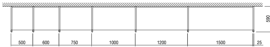
Larghezze moduli montante esterno Width of the modules with external upright
