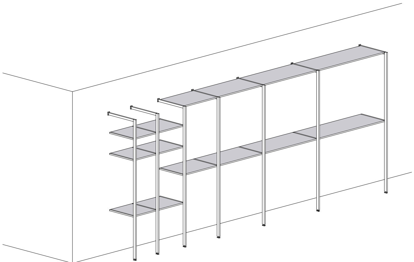
Altezze moduli Heights of the modules
