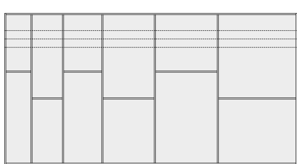
Altezze e prospetti moduli senza ante Modules without doors - height and front view
