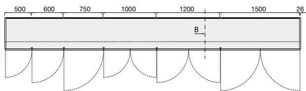
Larghezze moduli con montante interno Widths of internal upright modules
