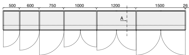
Larghezze moduli fianco legno Widths of wooden side modules
