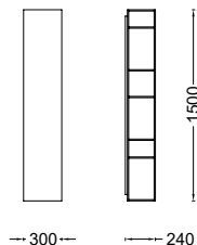
Elemento pensile \ Hanging element
