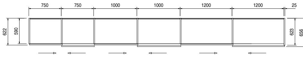
Larghezze moduli fianco legno Width of the modules with wooden side
