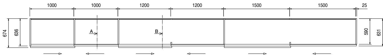
Larghezze moduli fianco legno/montante interno Width of the modules with wooden side/internal upright
