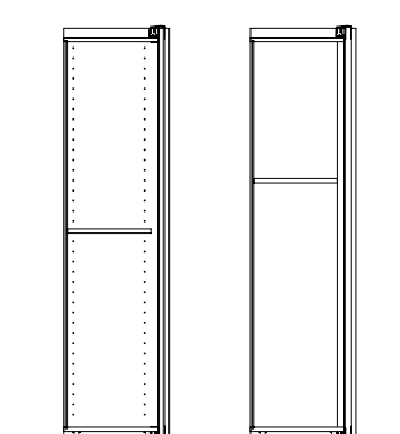
Sezione A Section A
