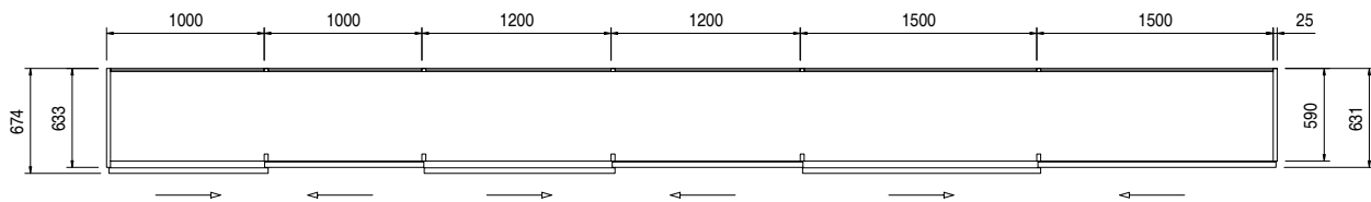
Larghezze moduli montante interno Width of the modules with internal upright
