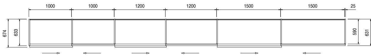
Larghezze moduli fianco legno Width of the modules with wooden side
