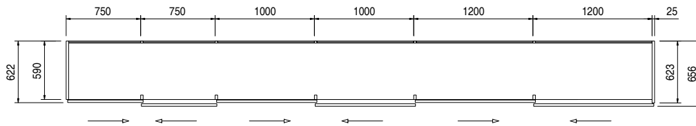
Larghezze moduli montante interno Width of the modules with internal upright
