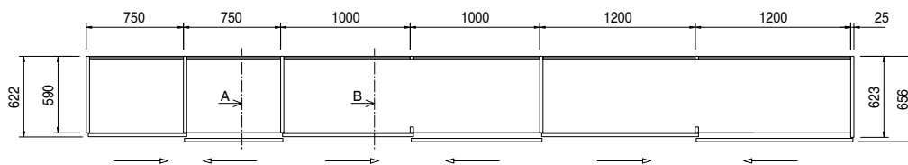
Larghezze moduli fianco legno/montante interno Width of the modules with wooden side/internal upright
