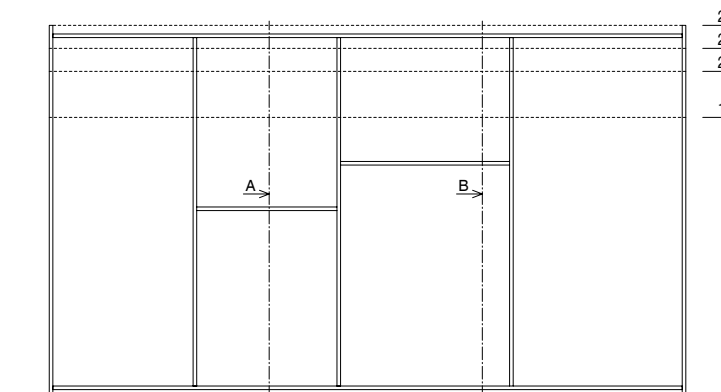
Altezze moduli senza ante Height of the modules without doors
